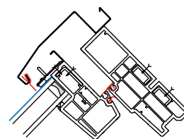
Dwarsdoorsnede raam en kaderprofiel
